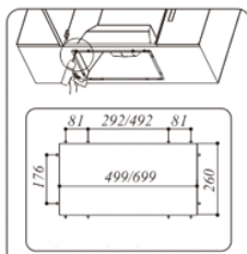
miejsca montażowe 12 śrub
